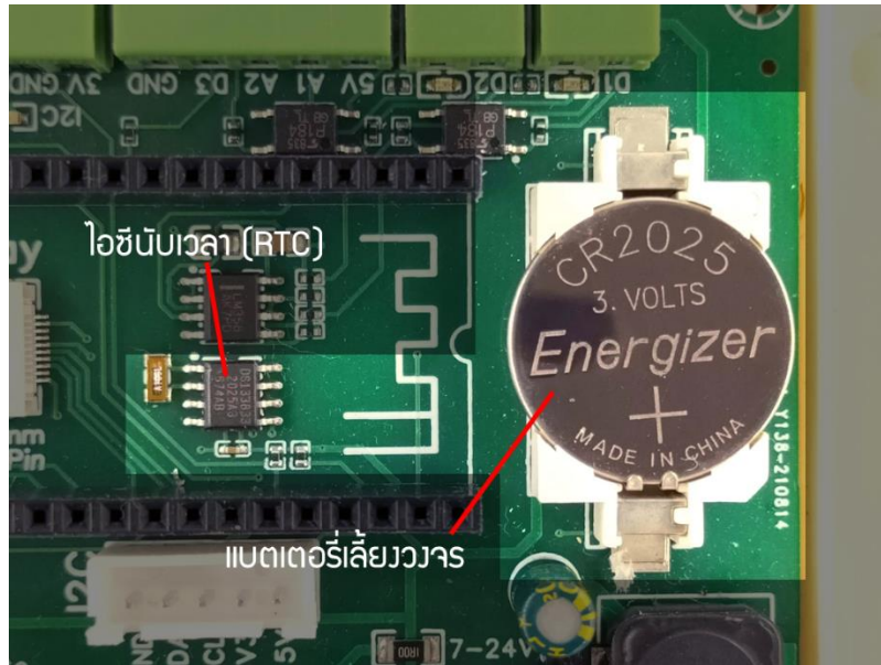
รูปที่ 23 ส่วนประกอบวงจรนับเวลา (RTC)
