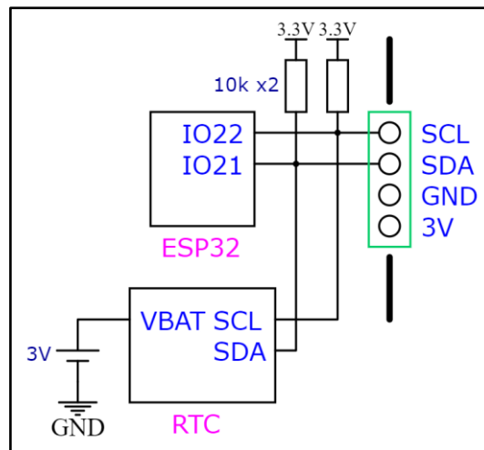
รูปที่ 24 บล็อกไดอะแกรมส่วนวงจรนับเวลา (RTC)
